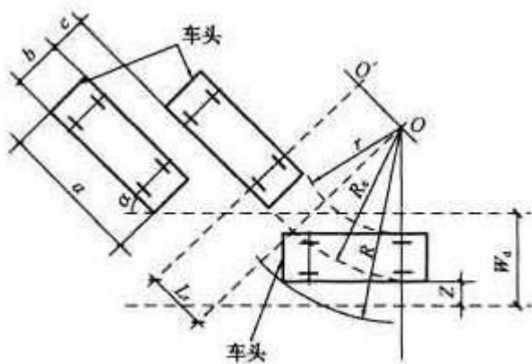
图15 前进停车平面
