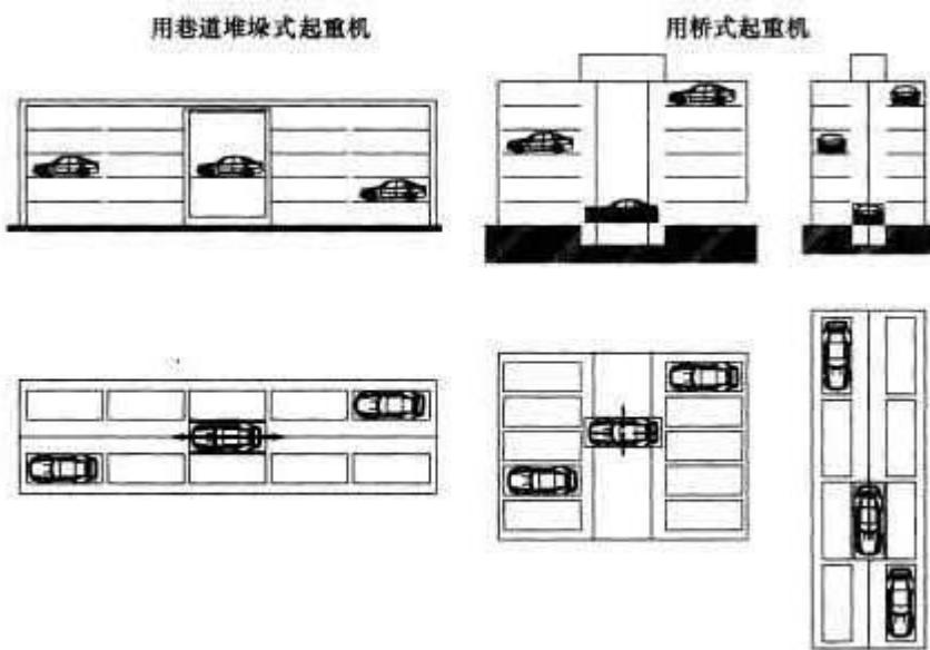
图6 巷道堆垛类停车设备示意图
