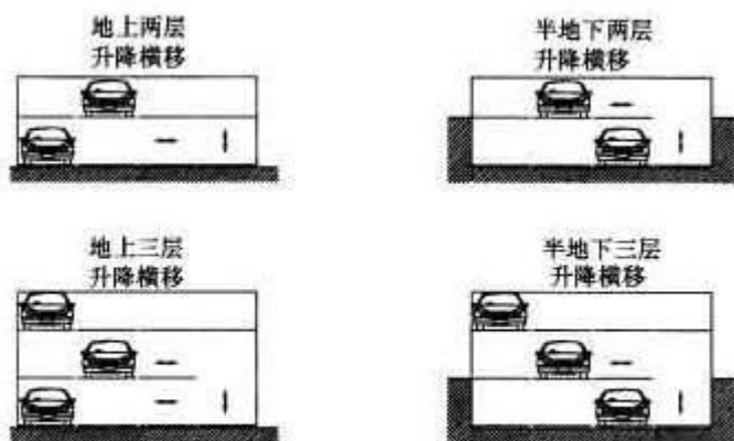
图1 升降横移类停车设备示意图
