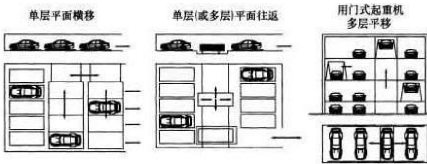
图5 平面移动类停车设备示意图
