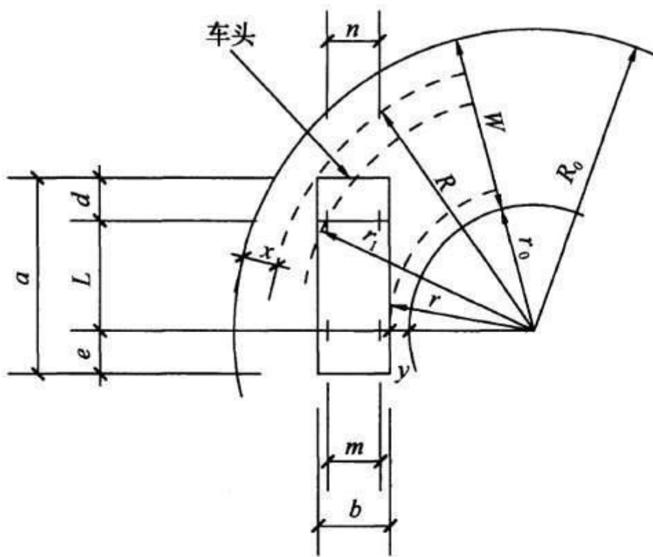
图 4.1.4 机动车环形车道平面图
