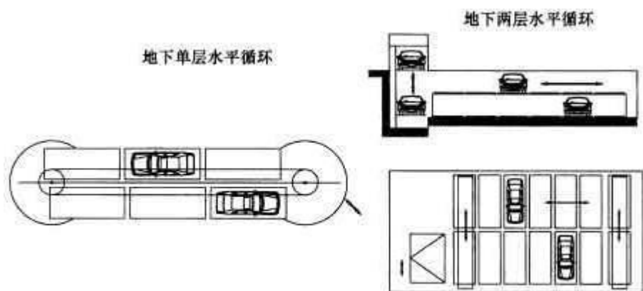
图3 水平循环类停车设备示意图
