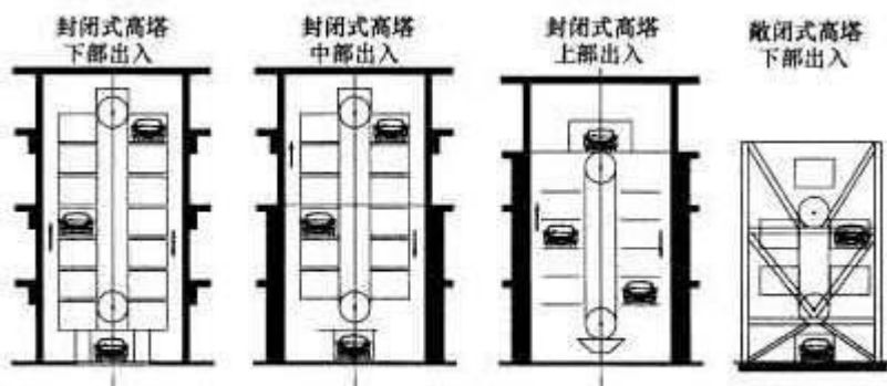
图2 垂直循环类停车设备示意图
