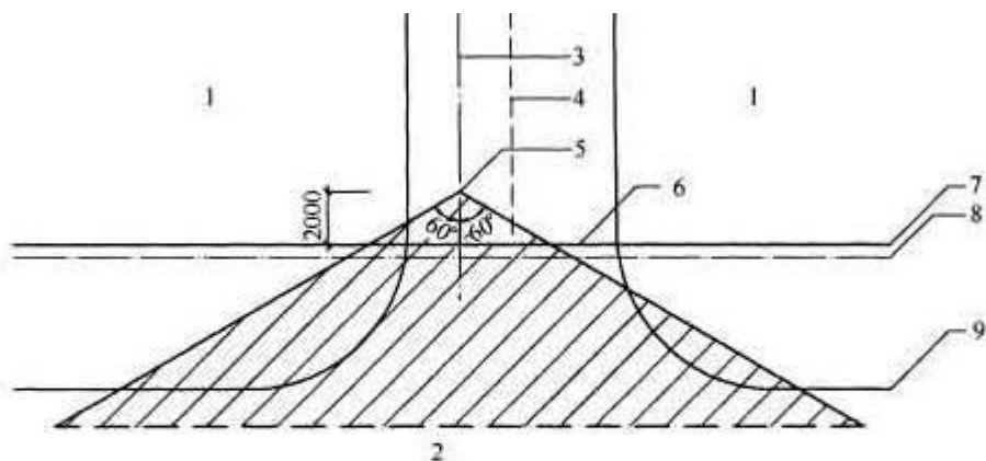
图9 机动车基地出入口通视要求示意图
