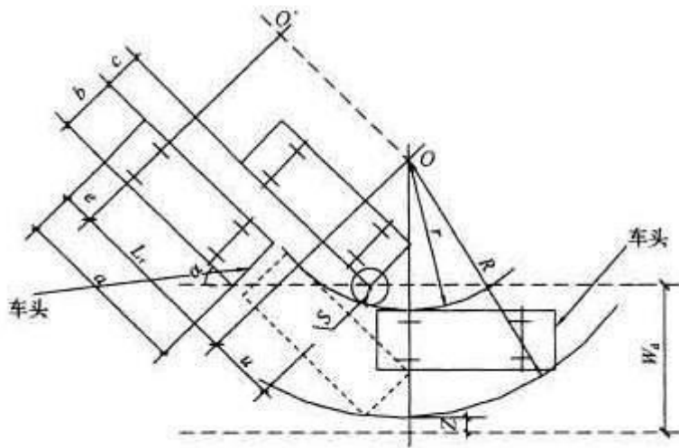
图16 退后停车平面
