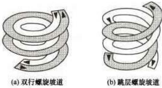
图13 双行和跳层螺旋坡道
