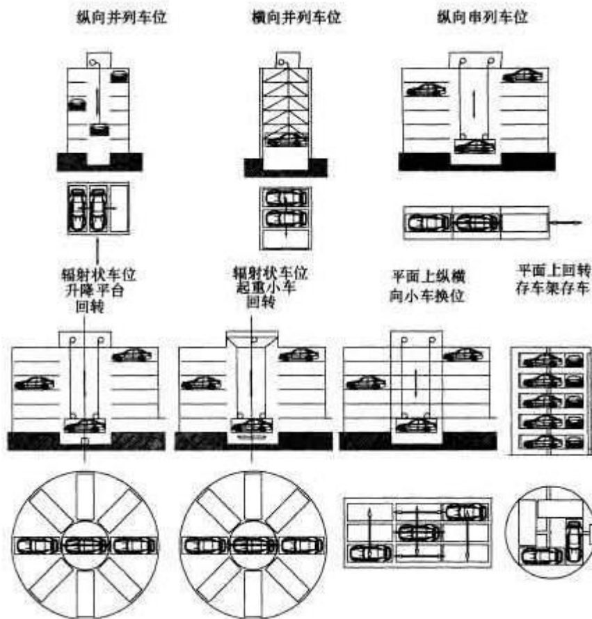
图7 垂直升降类停车设备示意图
