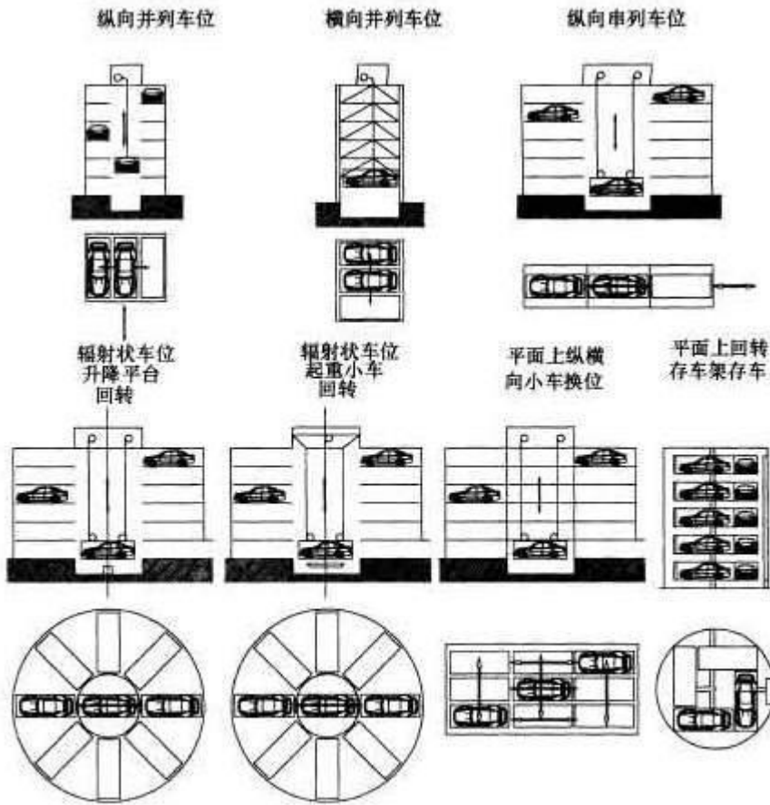
图8 简易升降类停车设备示意图
