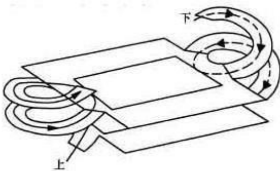
图12 单螺旋坡道式机动车库
