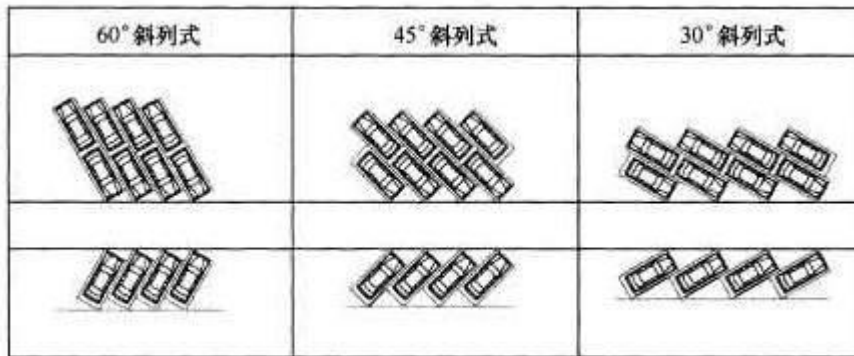
图14 斜列式停车方式的可能性布局
