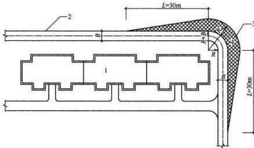
图10 场地内消防车道的弯道设计示意图
