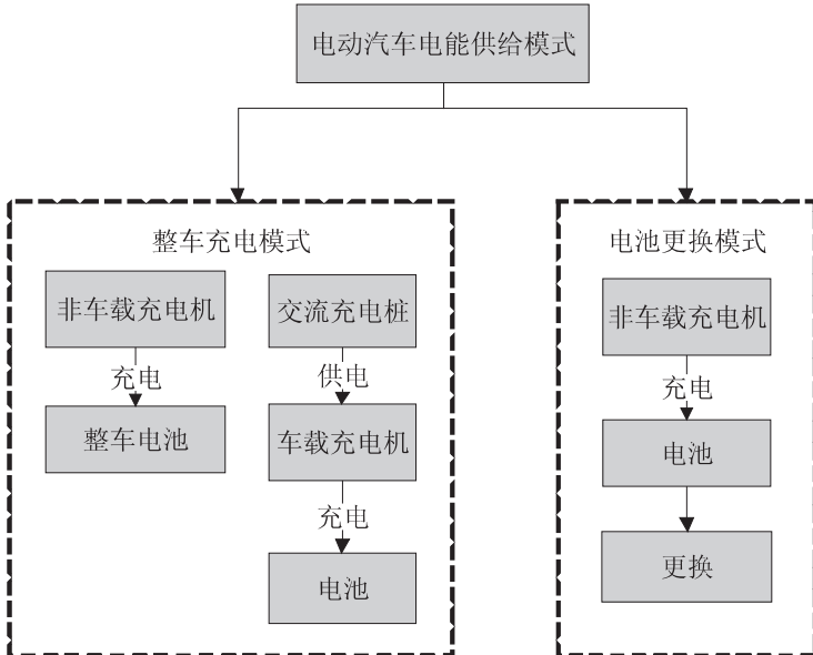
图 2.0.19 电动汽车电能供给模式
